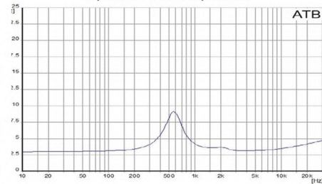
Impedanzverlauf / Impedance
